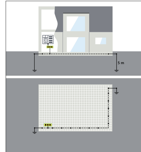
Stab-/Tiefenerder
