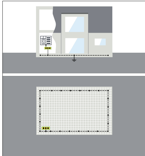
Fundamenterder
