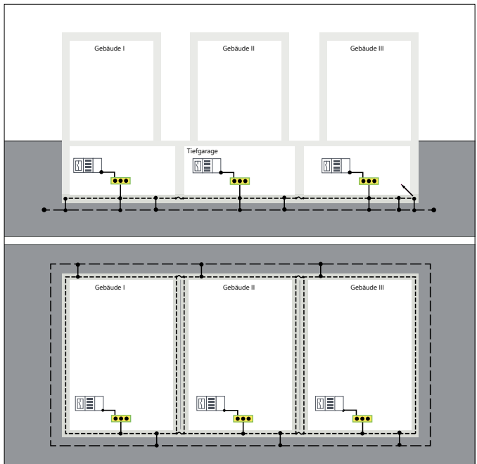
Erdungsanlage mit Ringerder und CBN für Mehrfamilienhaus
