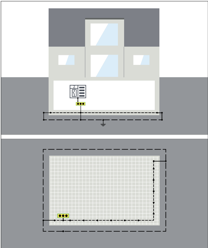
Erdungsanlage mit Ringerder für Wohngebäude mit Keller
