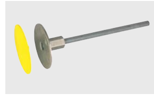
Erdungsfestpunkt Typ M Art.-Nr. 478 011 Durchmesser: 10 mm Anschlussachse: l = 180 mm Anschlussgewinde: M10/M12
