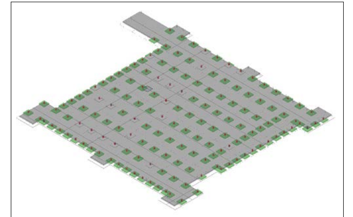
Gesamtansicht einer Erdungsanlagen Industrie mit Einzel- / Punktfundamenten
