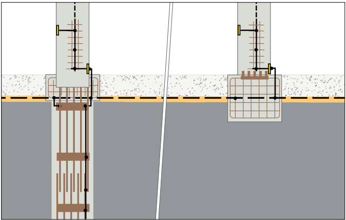
Bautechnische Ausführung von Einzelfundamenten
