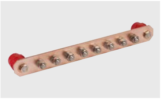
Potentialausgleichsschiene Industrie Art.-Nr. 472 227 Werkstoff: Cu Anzahl Anschlüsse: 8
