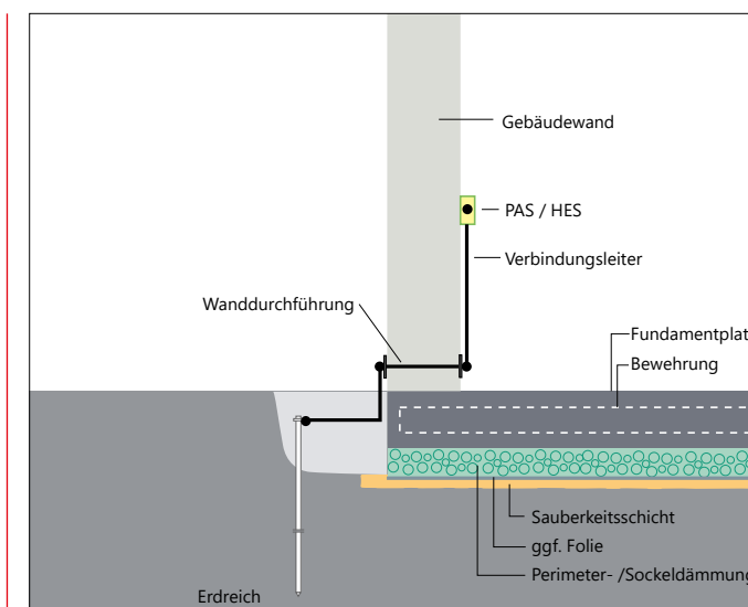
Praktische Ausführung Tiefererder ohne Keller
