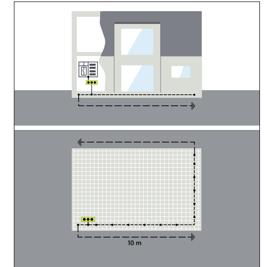
Strahlenerder
