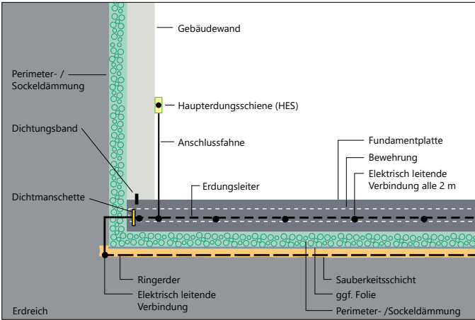
Praktische Ausführung mit Ringerder
