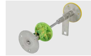
Wanddurchführung mit Druckwasserschutz Art.-Nr. 478 540 Werkstoff: NIRO (V4A) Anschlussgewinde: M10/M12
