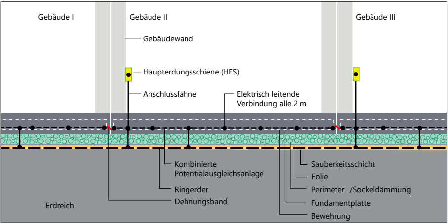
Praktische Ausführung Ringerder und CBN
