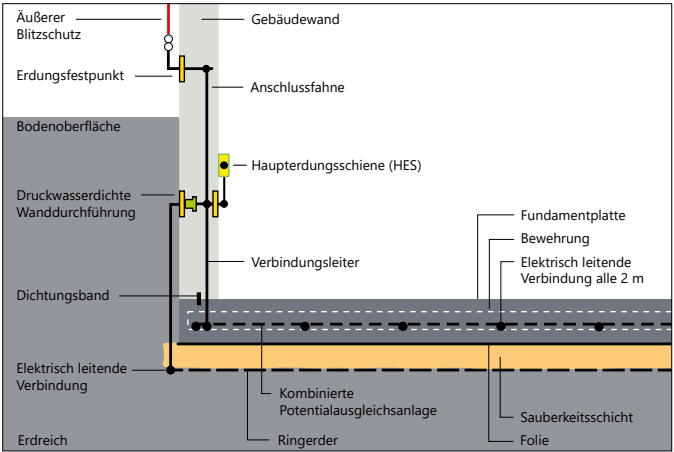
Praktische Ausführung Ringerder und CBN
